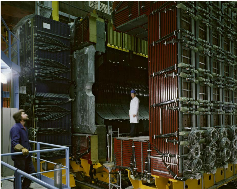
UA1
