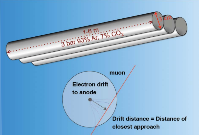
ATLAS : spectromètre \mu
