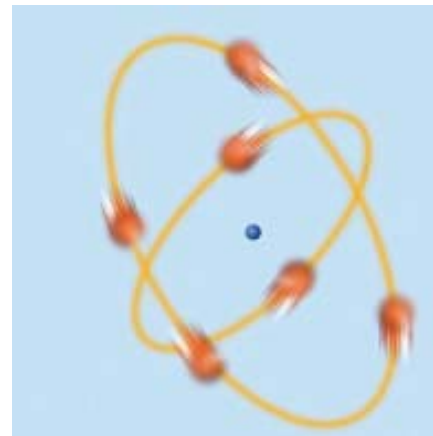
Bohr (1913)
