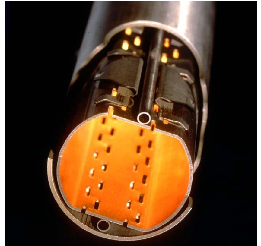
chambre à vide du LHC (en coupe)
