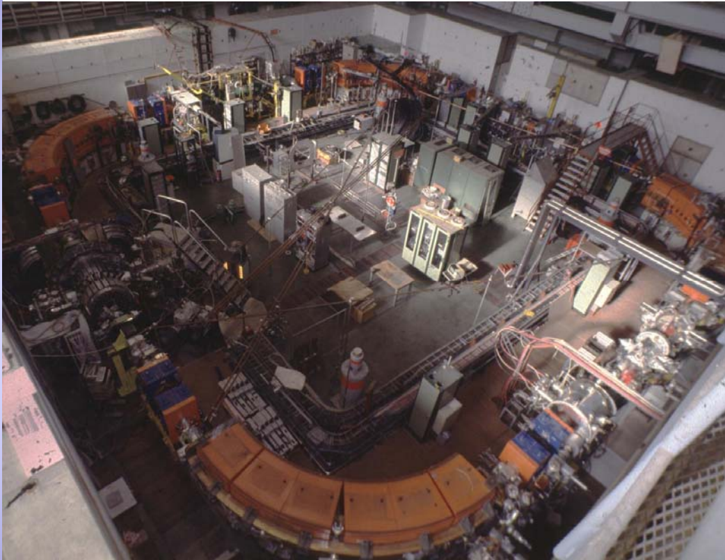
L'anneau LEAR d'antiprotons à basse énergie
